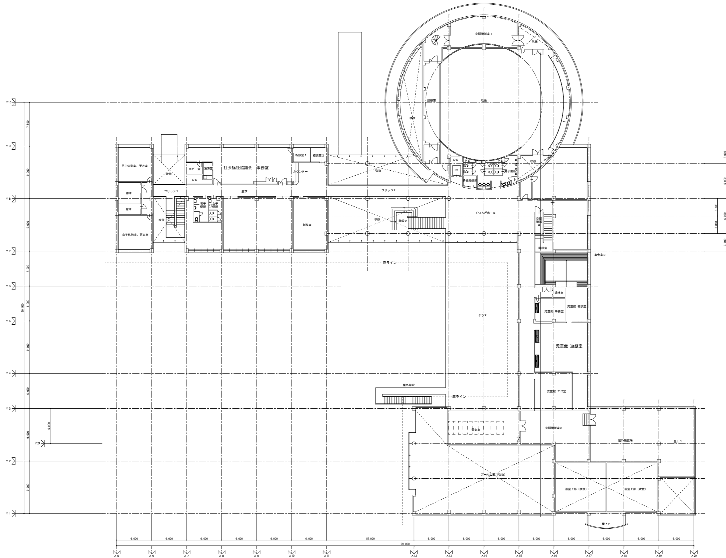
全体2階平面図 S=1/200
