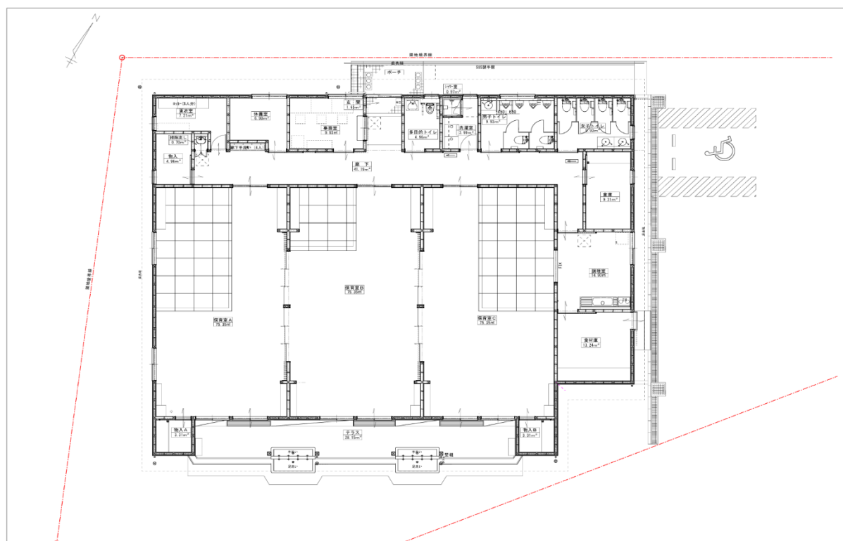
平面図
