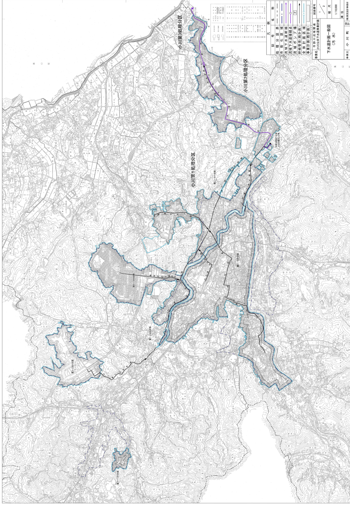
図 3.3.1 下水道計画一般図（污水、令和6年度提出）
