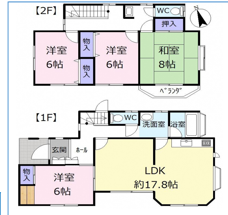
【間取図】
