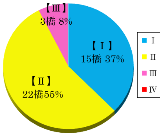
図-1 点検結果による判定区分
