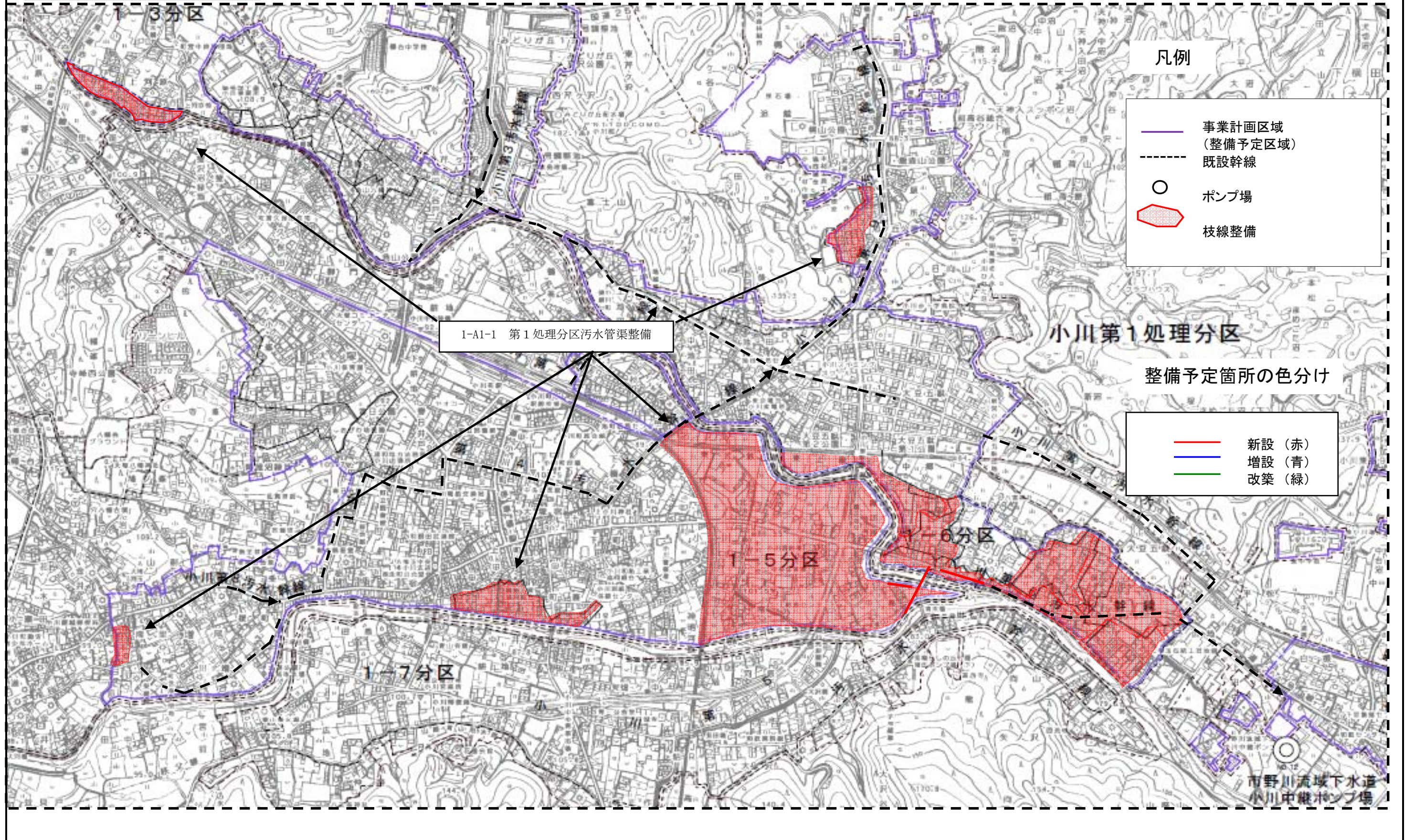
小川第1処理分区計画図
